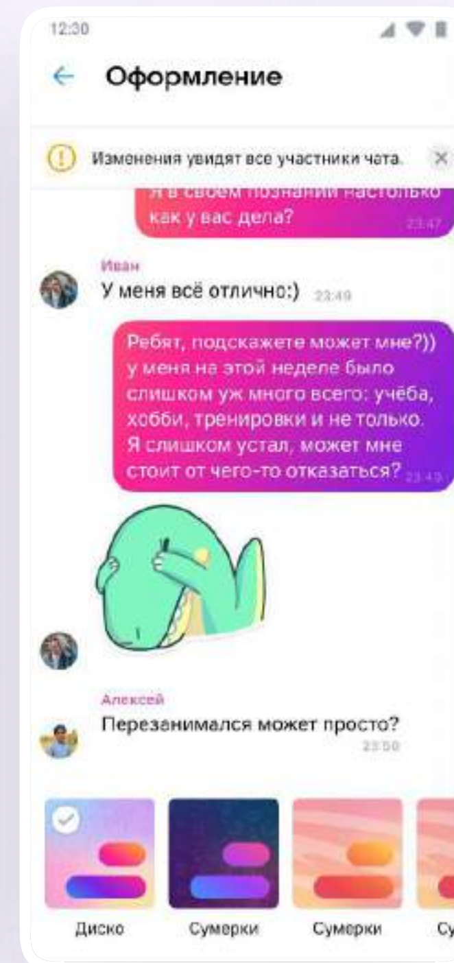
Android
